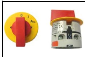
Interruttore avviamento starting switch CODICE/CODE: 2191 V 230 - 12 A
